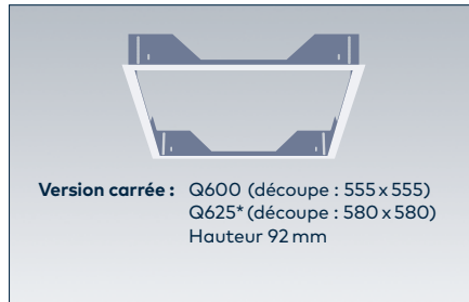
KIT POUR PLACOPLÂTRE
